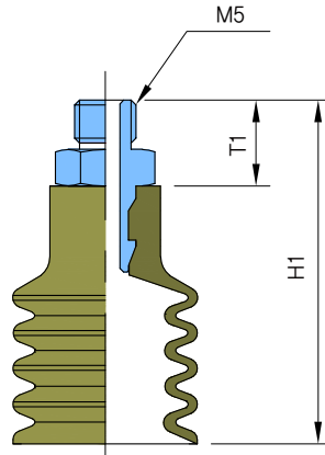
▶ 연결나사 조립도(숫나사)
