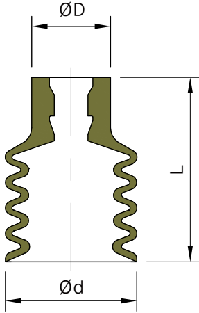
▶ 패드 외형도
