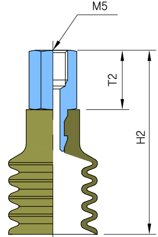
▶ 연결나사 조립도(암나사)
